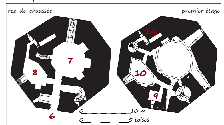
Plans du rez-de-chaussée et du premier étage du donjon
