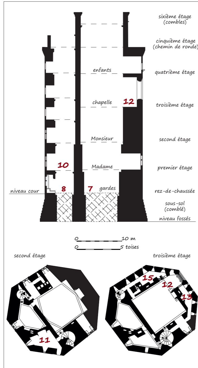
Coupe et plans des second et troisième étages du donjon
